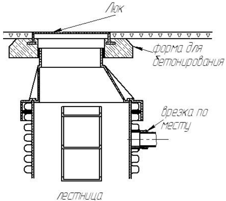
Схема сборки колодца и установки люка
